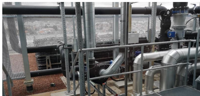
Abbildung 3: Anlagentechnik am Dach, mit Solarabsorbern im Hintergrund (Quelle: AEE INTEC)
