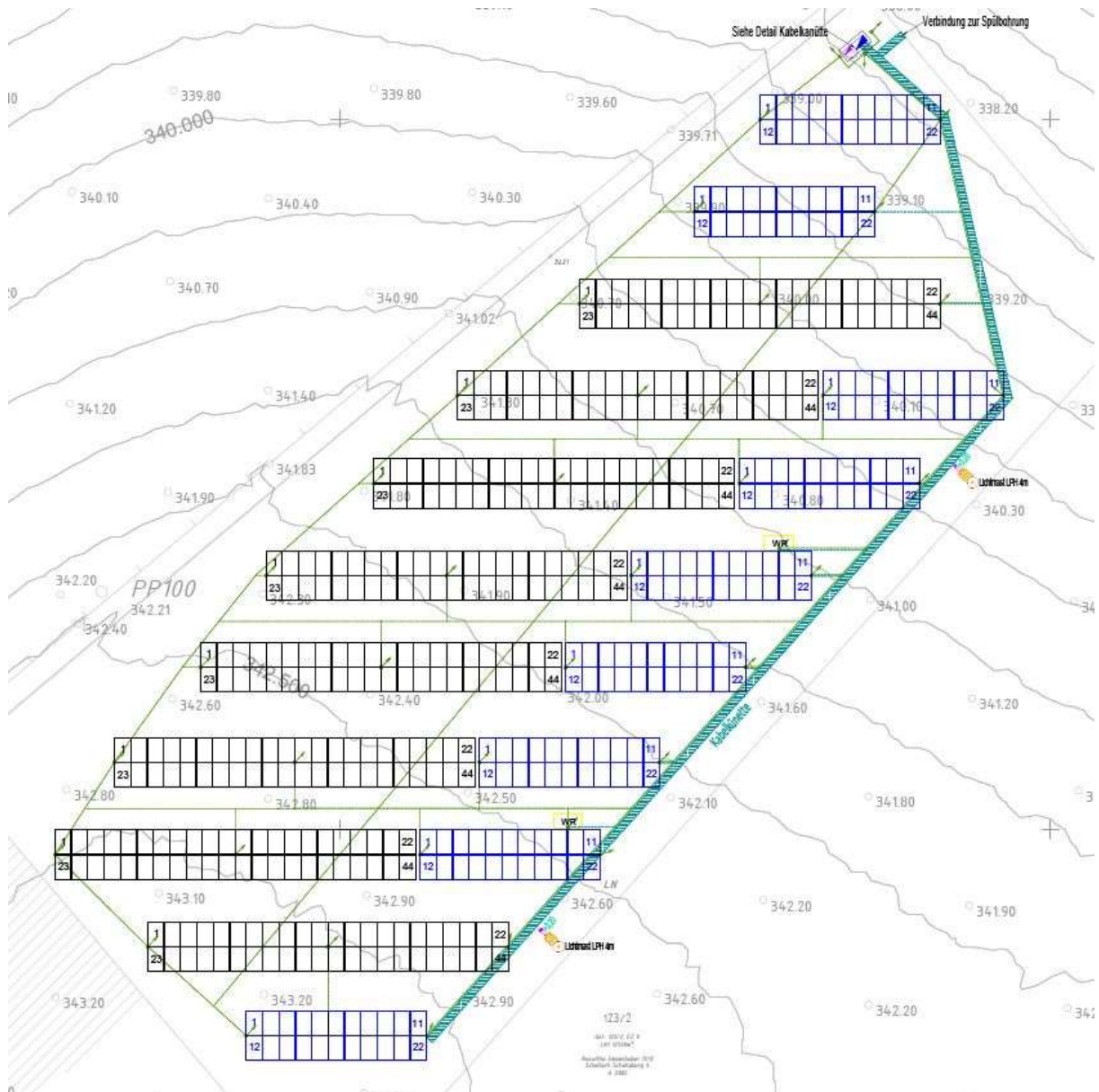
Bild1, Grundrissplan der geplanten PV-Freiflächenanlage
