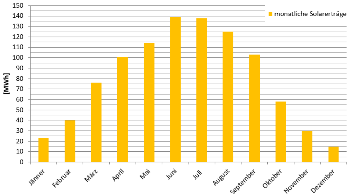
Abbildung 2: Monatliche Ertragsprognose für das Solarsystem
