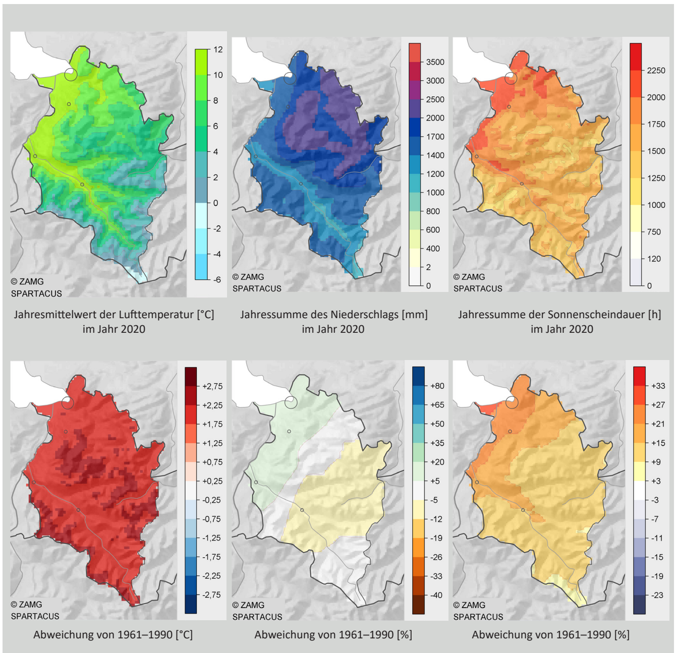
Abbildung 3: Räumliche Verteilung der Jahreswerte 2020 von Lufttemperatur (links), Niederschlagssumme (Mitte) und Sonnenscheindauer (rechts) in Vorarlberg als Absolutwerte (oben) und als Abweichungen vom Mittelwert des Bezugszeitraumes 1961–1990 (unten).
