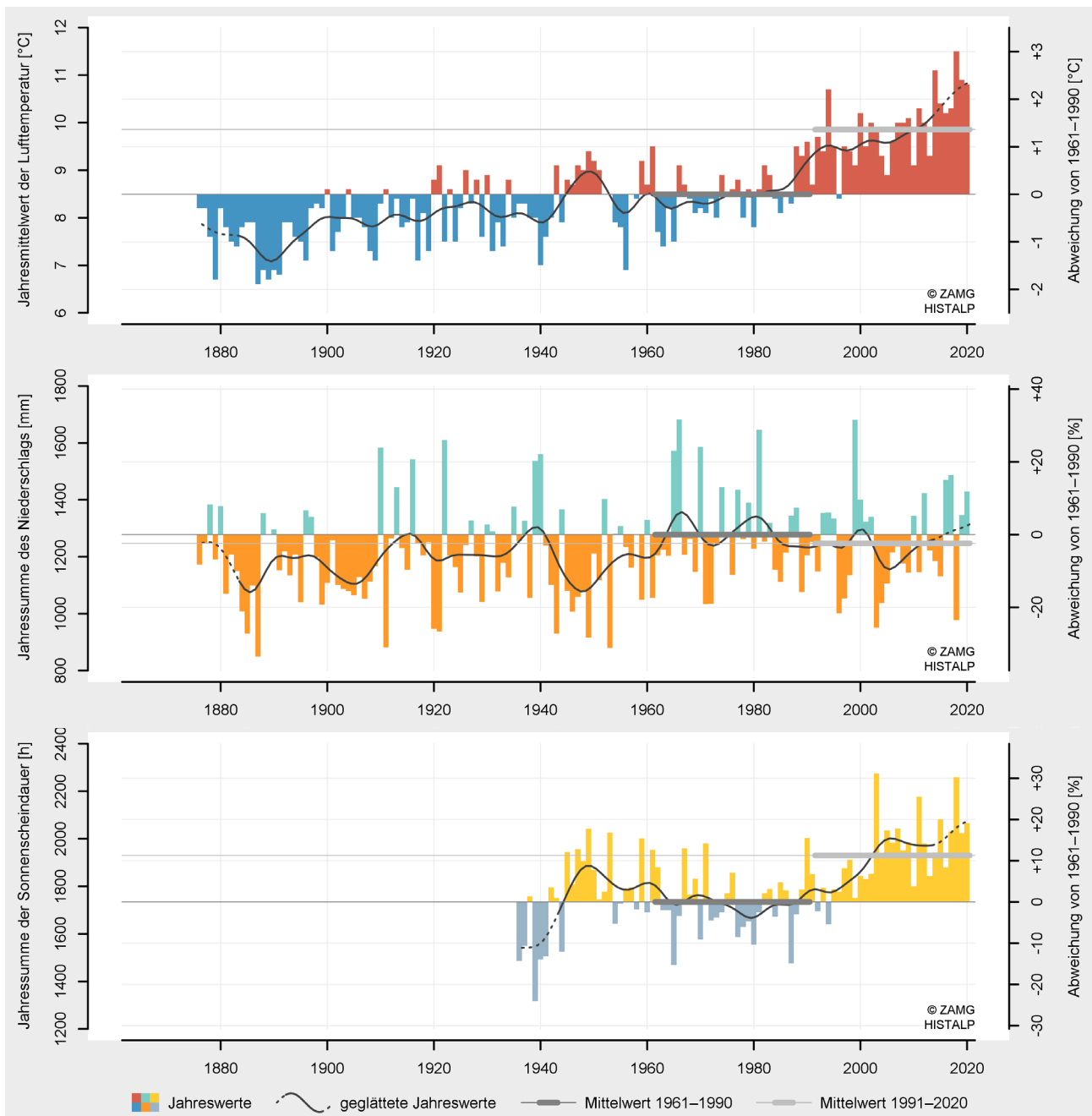
Abbildung 4: Langfristige Entwicklung der Jahreswerte von Lufttemperatur (oben), Niederschlagssumme (Mitte) und Sonnenscheindauer (unten) in Feldkirch vom Beginn instrumenteller Messungen bis 2020. Die Niveaus der Mittelwerte des Bezugszeitraumes 1961–1990 bzw. der letzten 30 Jahre 1991–2020 sind als dunkelgraue bzw. hellgraue horizontale Linien eingetragen.
